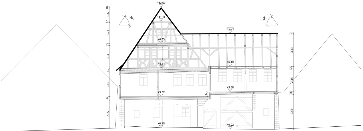
Schnitt
